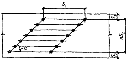
Рис. 12. Расстановка гвоздей косыми рядами
