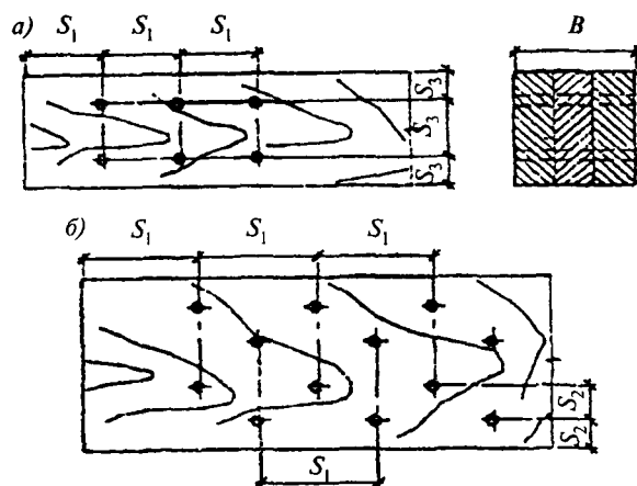
Рис. 10 Расстановка нагелей
