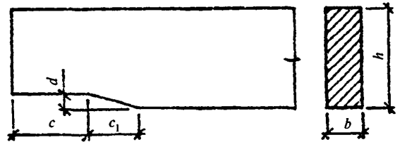
Рис. 15. Скошенная подрезка конца балки
