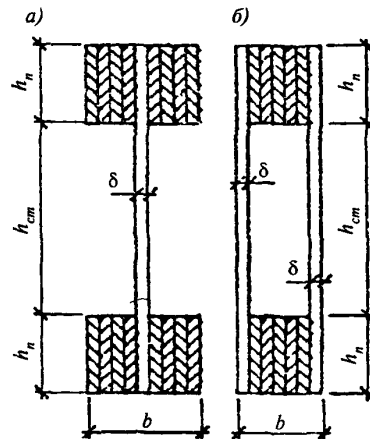
Рис. 4. Поперечное сечение клееных балок с плоской фанерной стенкой
