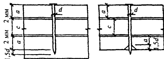
Рис. 11. Определение расчетной длины защемления конца гвоздя
