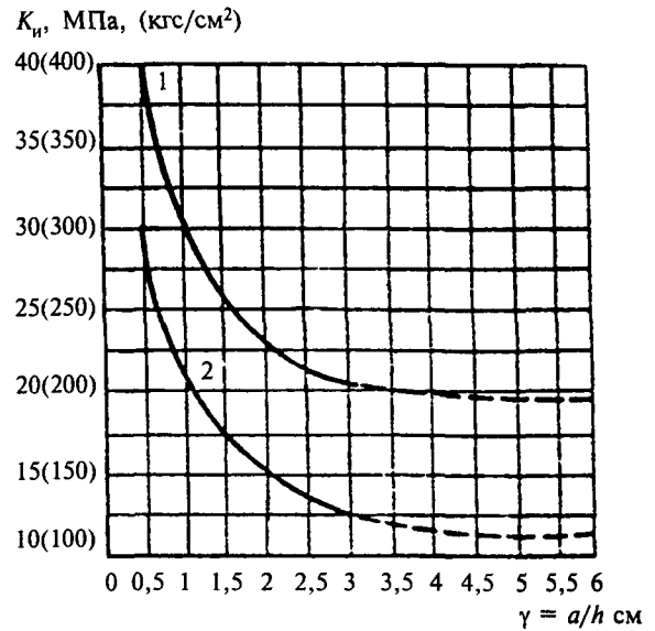
Рис. 2. Графики для определения коэффициента k_n при расположении волокон в наружных слоях фанеры вдоль пролета
