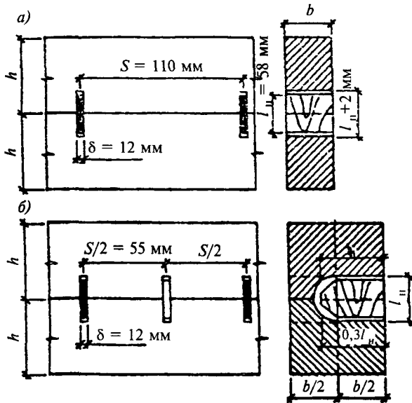
Рис. 13. Соединение на пластинчатых нагелях
