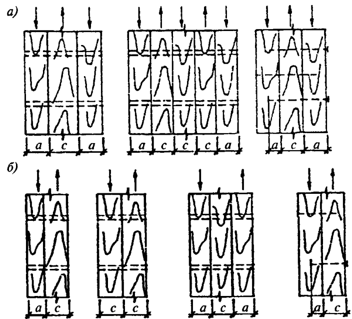
Рис. 8. Нагельные соединения
