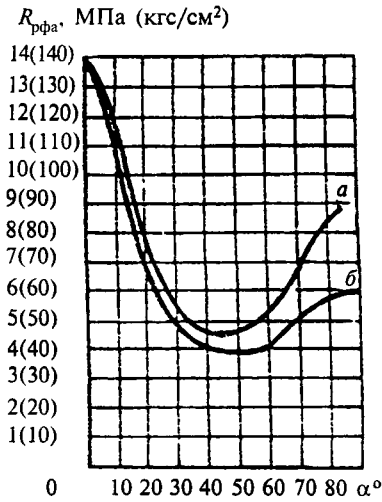
Рис. 1. Графики для определения расчетных сопротивлений при растяжении под углом \alpha к волокнам наружных слоев березовой фанеры марки ФСФ а — семислойной, б — пятислойной
