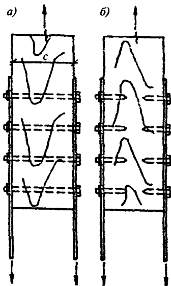
Рис. 9. Нагельные соединения со стальными накладками
