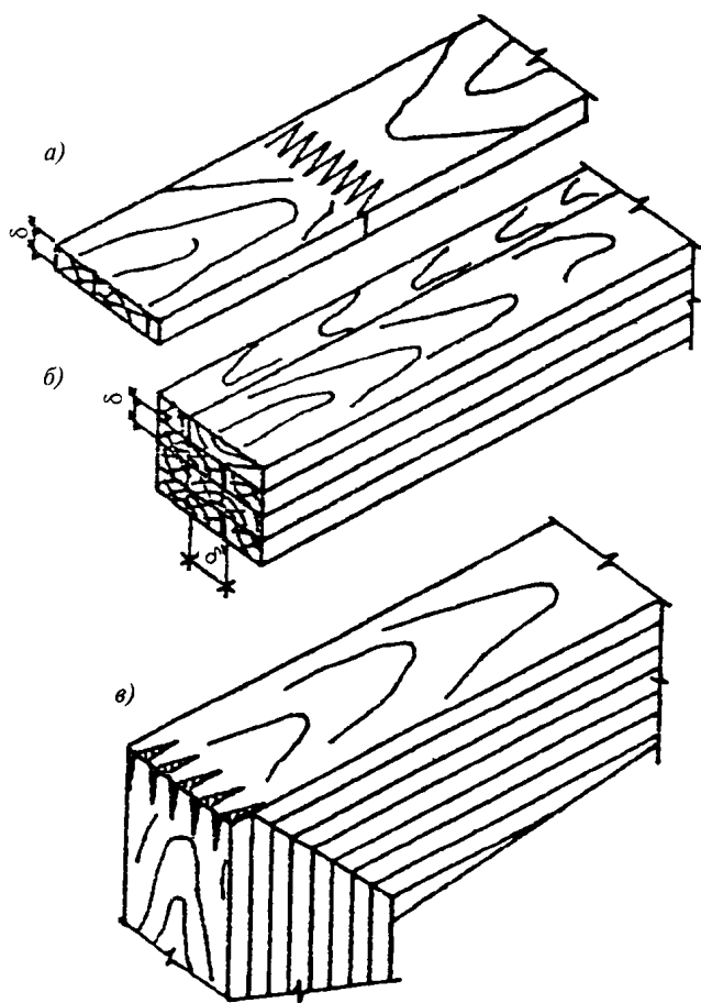
Рис. 6. Клеевые соединения
