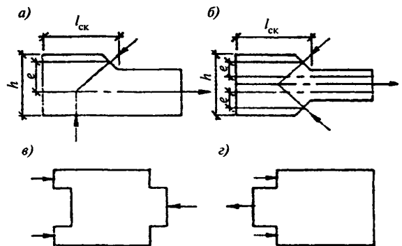
Рис. 5. Врезки в элементах соединений
